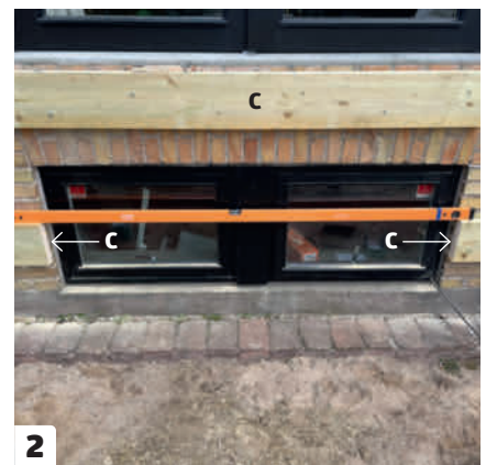
Asenna palkit (C) seinään. Alempi palkki kannattelee terassia, ylempi portaita. Poraa kansiruuveille valmiit reiät 6 millin kiviterällä ja kiinnitä palkki karmiruuveilla 30 sentin välein.
