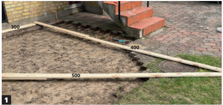
Mittaa terassin paikka ja viritä linjalangat kuten piirroksessa. Saat terassista suorakulmaisen, kun teet ison suorakulmaisen kolmion laudoista suhteessa 3:4:5. Tässä käytetään kolmiota, jonka sivut ovat 300, 400 ja 500 senttiä pitkät. Yksi kolmion kulmista on tarkasti 90 asteen kulmassa.
