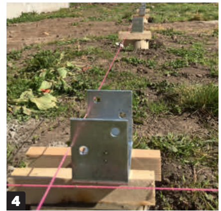
Upota tolppakengät märkään betoniin suoraan linjaan. Tue tolppakengät parilla laudanpötkällä betonin kuivumisen ajaksi.
