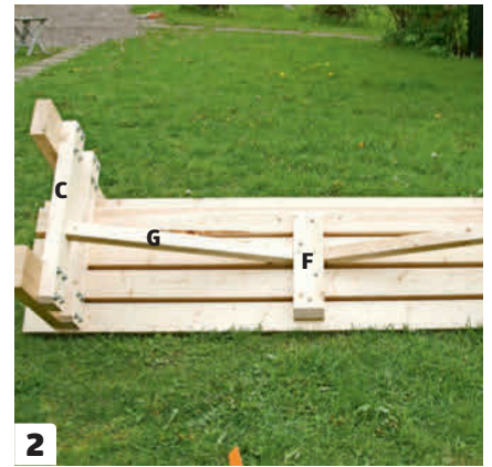
2 Kiinnitä vinotuet (G) lankunpätjän (F) ja päätyjen (C) väliin. Sahaa vinotukien päät sopivassa kulmassa ja ruuvaa ne kiinni 5x55 millin ruuveilla.
