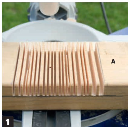
1 Poista lankusta puolet jalkojen (A) liitoskohdasta. Voit tehdä sen vanhanaikaisesti käsisahalla ja taltalla, mutta työ sujuu nopeammin sirkkelillä.
