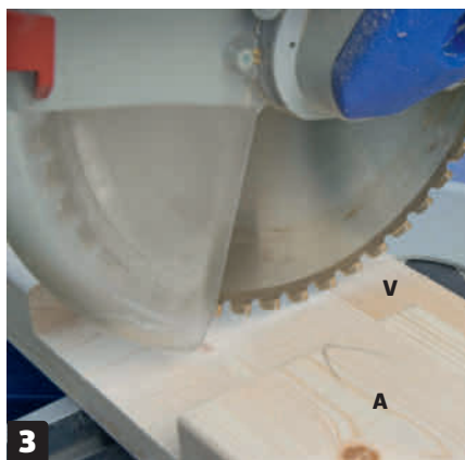
3 Siisti loven pohja sirkkelillä liikuttamalla lankkua terän alla. Käytä lankun ja sirkkelin ohjaimen välissä rimaa (V), jotta terä yltää loven pohjalle myös lankun takareunassa.
