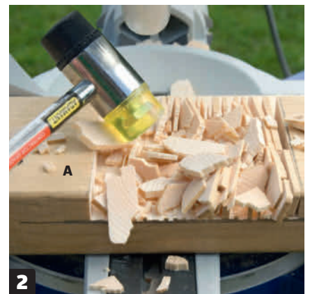
2 Sahaa puuhun paljon samansuuntaisia uria ja lyö niiden väliin jäävät suikaleet irti vasaralla.
