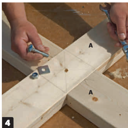
4 Yhdistä jalan osat pulteilla. Jalkojen (A) pitäisi sopia yhteen niin hyvin, että ne muodostavat suoran kulman. Osat yhdistetään pulteilla kuten penkin jalat. Tässä poranterä yltää kerralla puun läpi.
