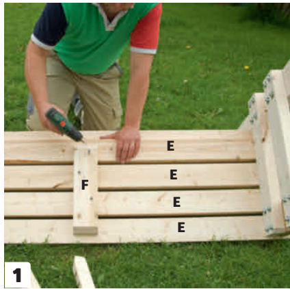
1 Asenna penkin keskelle poikkilankku (F). Ruuvaa se kiinni alapuolelta 6x80 millin ruuveilla. Asenna ruuvit vuorotellen eri reunoihin kuten kuvassa.
