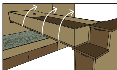
Den vendbare seng hviler på en liste monteret på bagvæggen mellem køjerne og på en MDF-plade i den anden ende.
