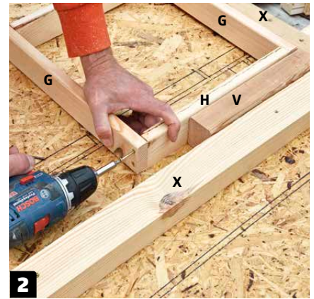
2 Kokoa laatikoiden rungot. Sivele liimaa kaikkiin liitoksiin, jotta laatikot kestävät mahdollisimman pitkään. Mahdut ruuvaamaan paremmin, jos kiinnität sapluunan kylkeen lyhyen lisäkapulan (V).
