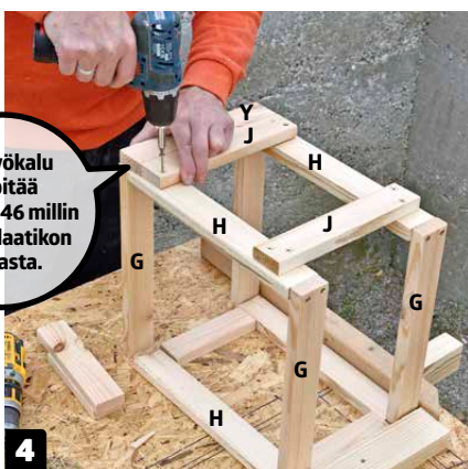
4 Kasaa laatikoiden reunat yhteen kahdella poikkirimalla (J). Rimat toimivat samalla laatikoiden kantokahvoina. 46 millillä leveä aputyökalu pitää rimaa etäisyyden reunasta vakiona.
