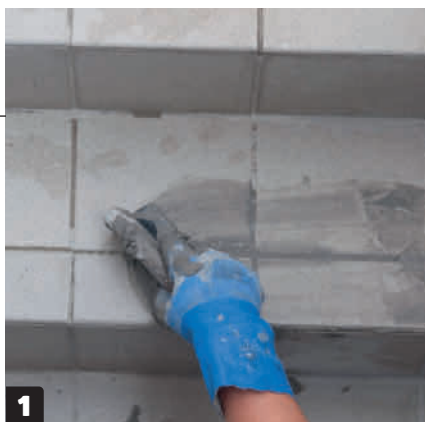
1 Trekk på fugemasse med en fugesparkel. Trekk den diagonalt over fugene, slik at fugemassen presses godt ned i dem.
