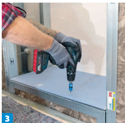
3 Asenna levyt runkoon kipsiruuveilla. Upota ruuvit hieman levyn pinnan alle. Voit käyttää syvyysrajoitinta, jotta ruuvit eivät mene liian syvälle.
