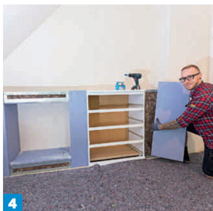
4 Asenna kipsilevyt joka puolelle, jotta eristeet eivät jää näkyviin.
