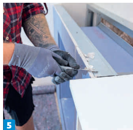
5 Leikkaa levyjen reunat suoriksi. Voit vetää terää teräsrankaa pitkin.
